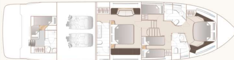
F65 Layout des Unterdecks
